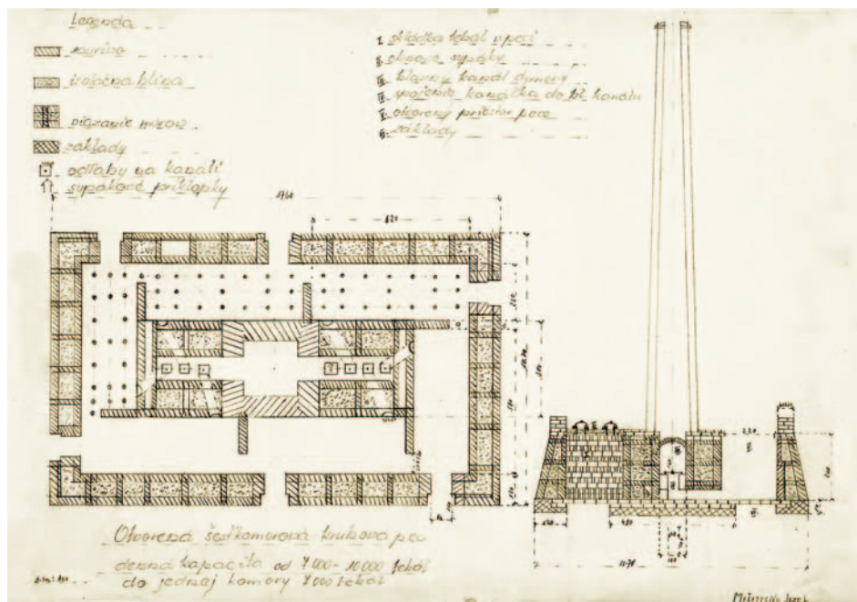
Druhý plán od Jozefa Mišínského, nedatováno – rok 1967 (?) (soukromá sbírka Stanislava Schneidera)
