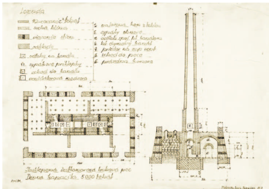
První, nekolorovaný plán bývalé bulharské kruhové cihelny od Jozefa Mišínského z roku 1967 (soukromá sbírka Stanislava Schneidera)
