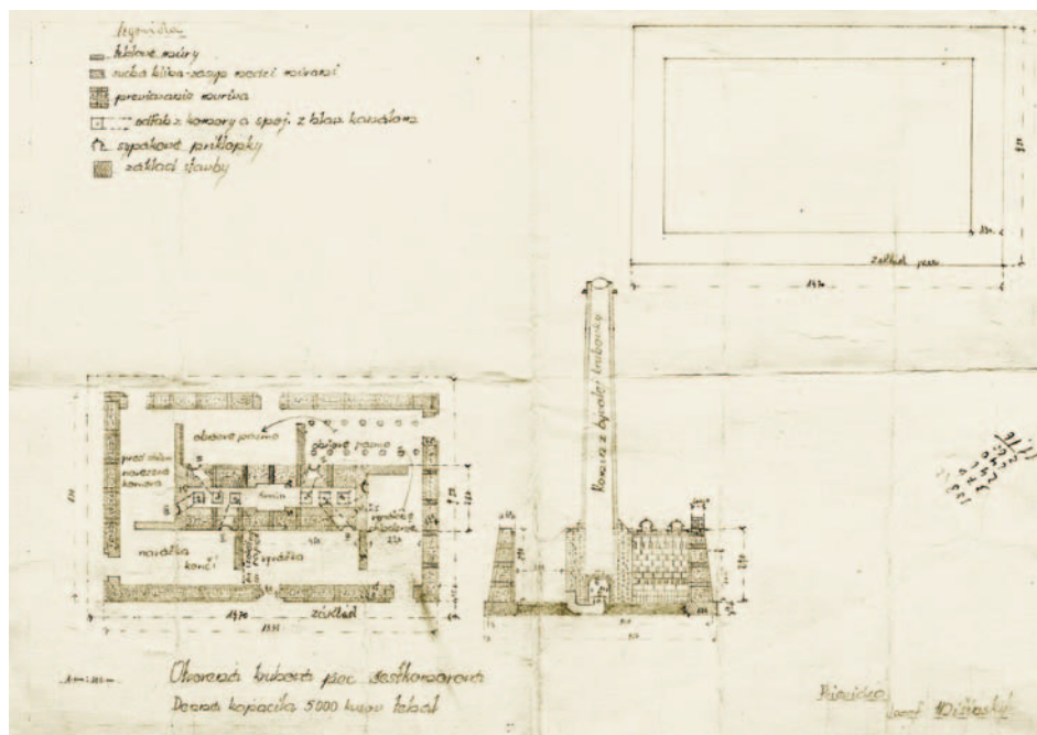
Třetí plán od Jozefa Mišínského, nedatováno – rok 1967 (?) (soukromá sbírka Stanislava Schneidera)
